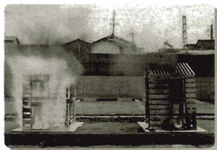
(左)無処理、(右)難燃防火処理
